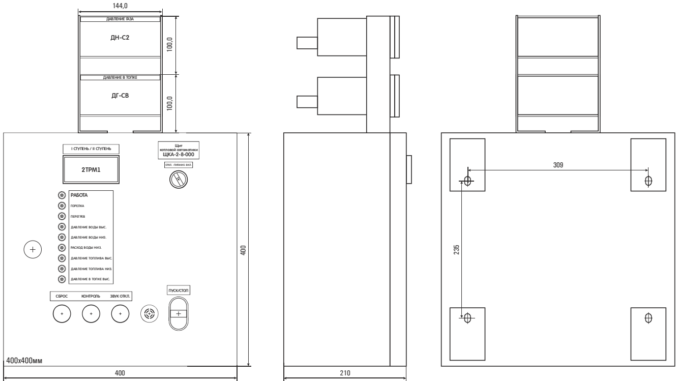
Рис.1. Внешний вид, габаритные и установочные размеры комплекта ЩКА-2-8-000/ЩКА-2-8-000К. В модификациях ЩКА-М-8-000/ЩКА-М-8-000К вместо 2TRM1 (I СТУПЕНЬ / II СТУПЕНЬ) установлен TRM12 (РЕГУЛИРОВАНИЕ).
